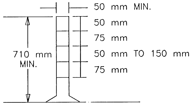
TUBULAR MARKERS
