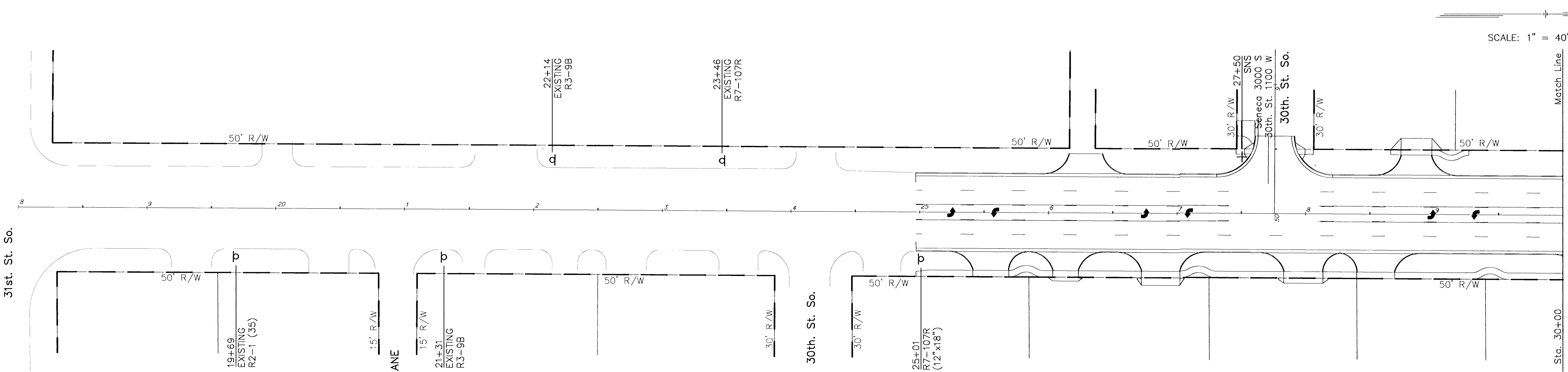
SENECA STREET - STA. 18+00 TO STA. 30+00
