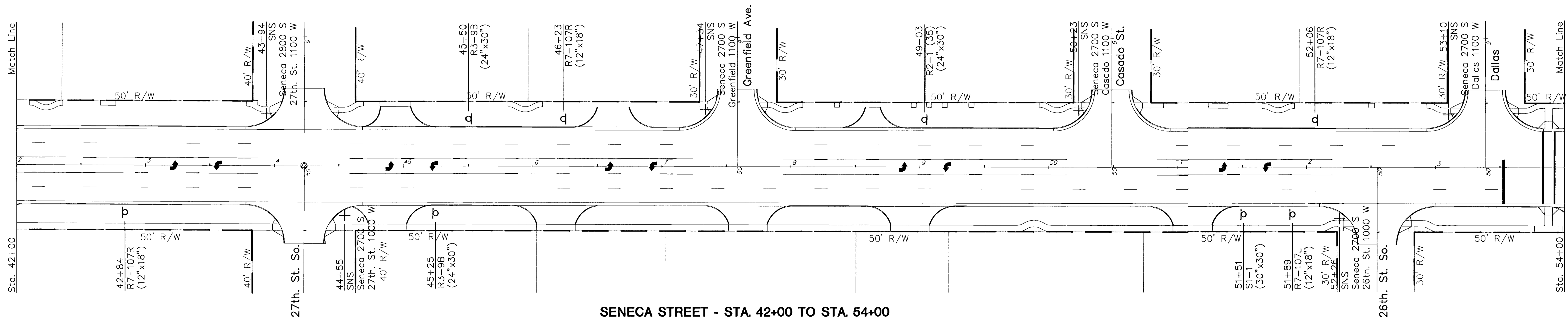
SENECA STREET - STA. 42+00 TO STA. 54+00
