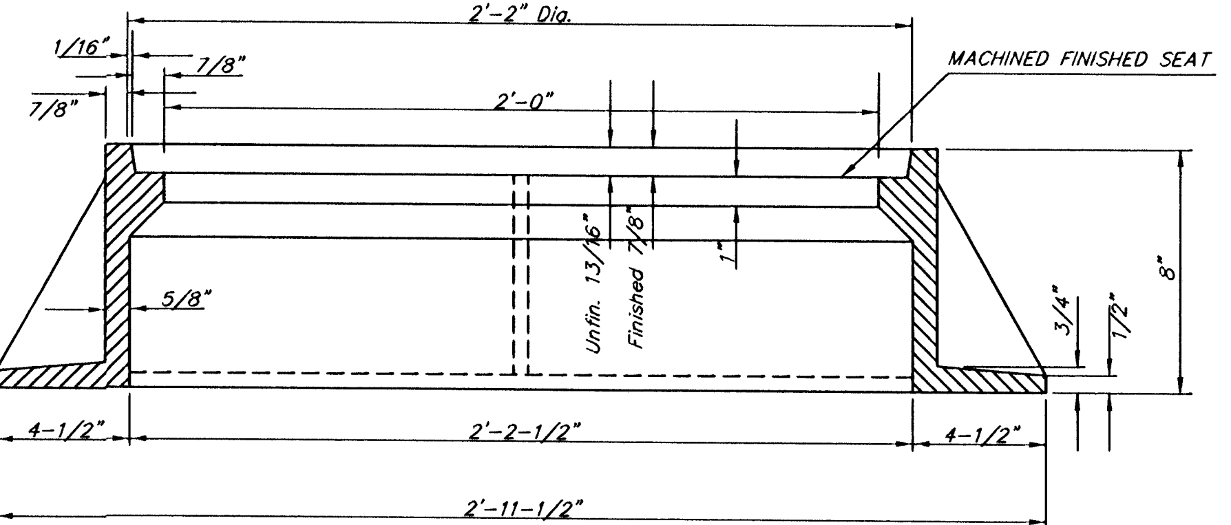
SECTION A-A
