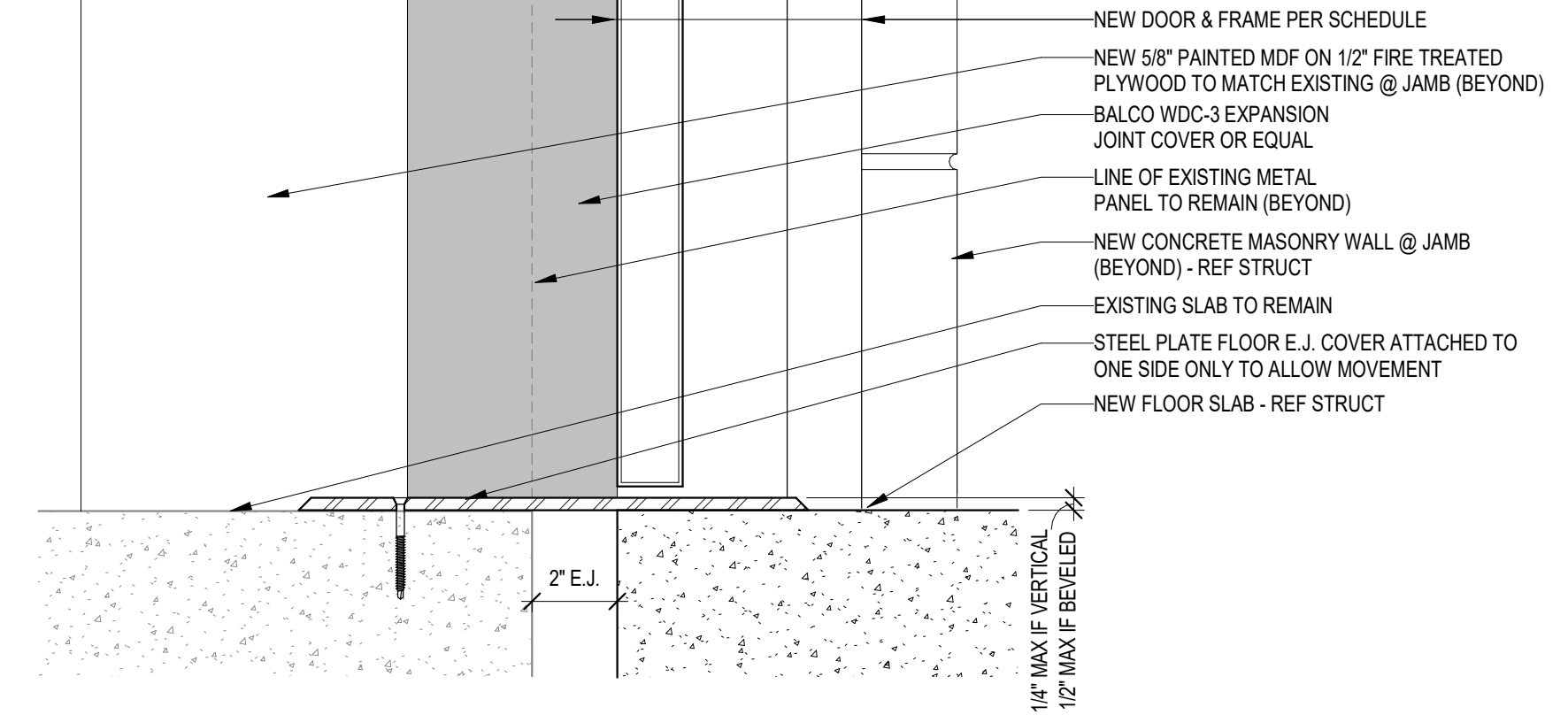
15 DOOR SILL @ EJ 3\"/>
