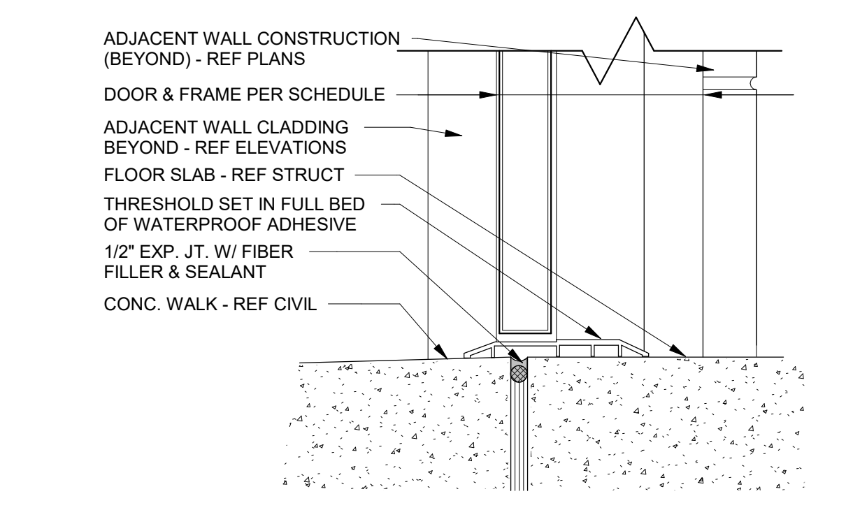
14 TYP THRESHOLD DETAIL 3\"/>
