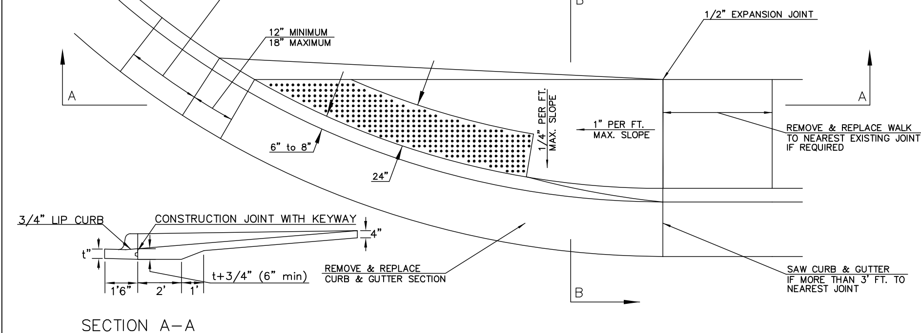
SECTION A-A
