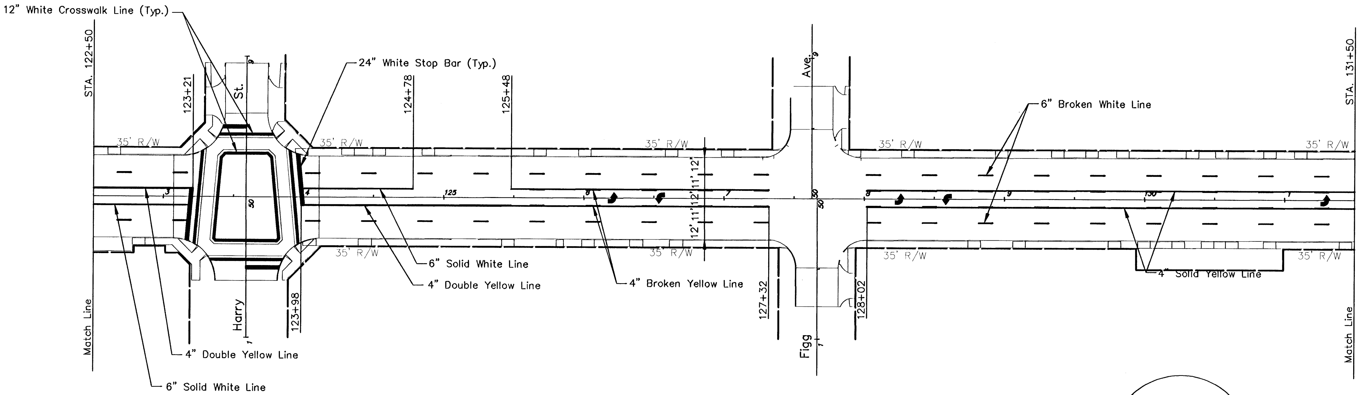
SENECA STREET - STA 122+50 TO STA 131+50
