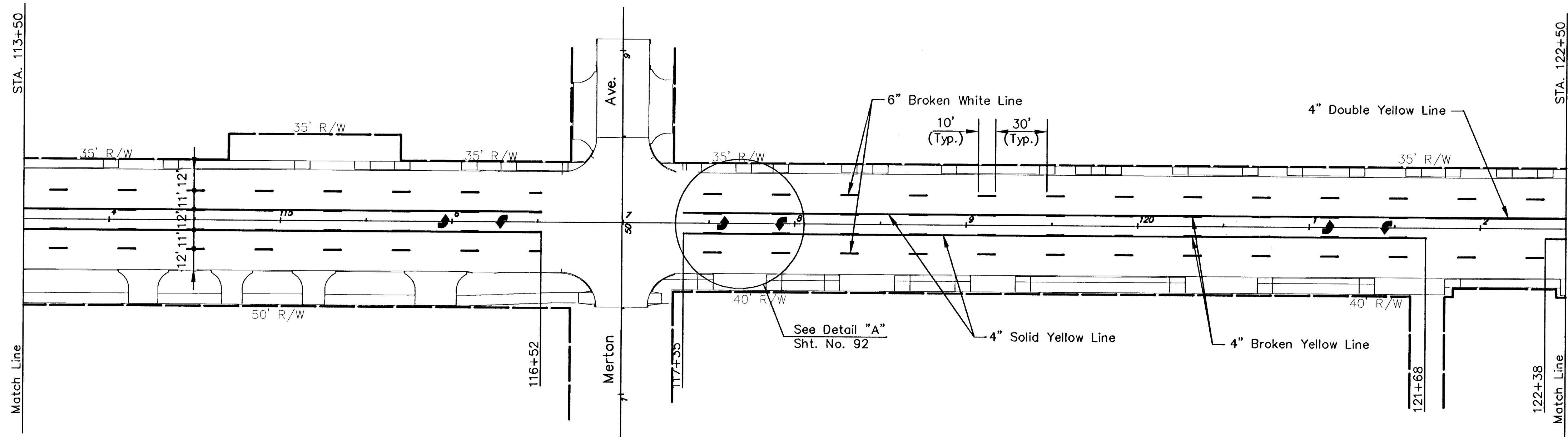
SENECA STREET - STA 113+50 TO STA 122+50
