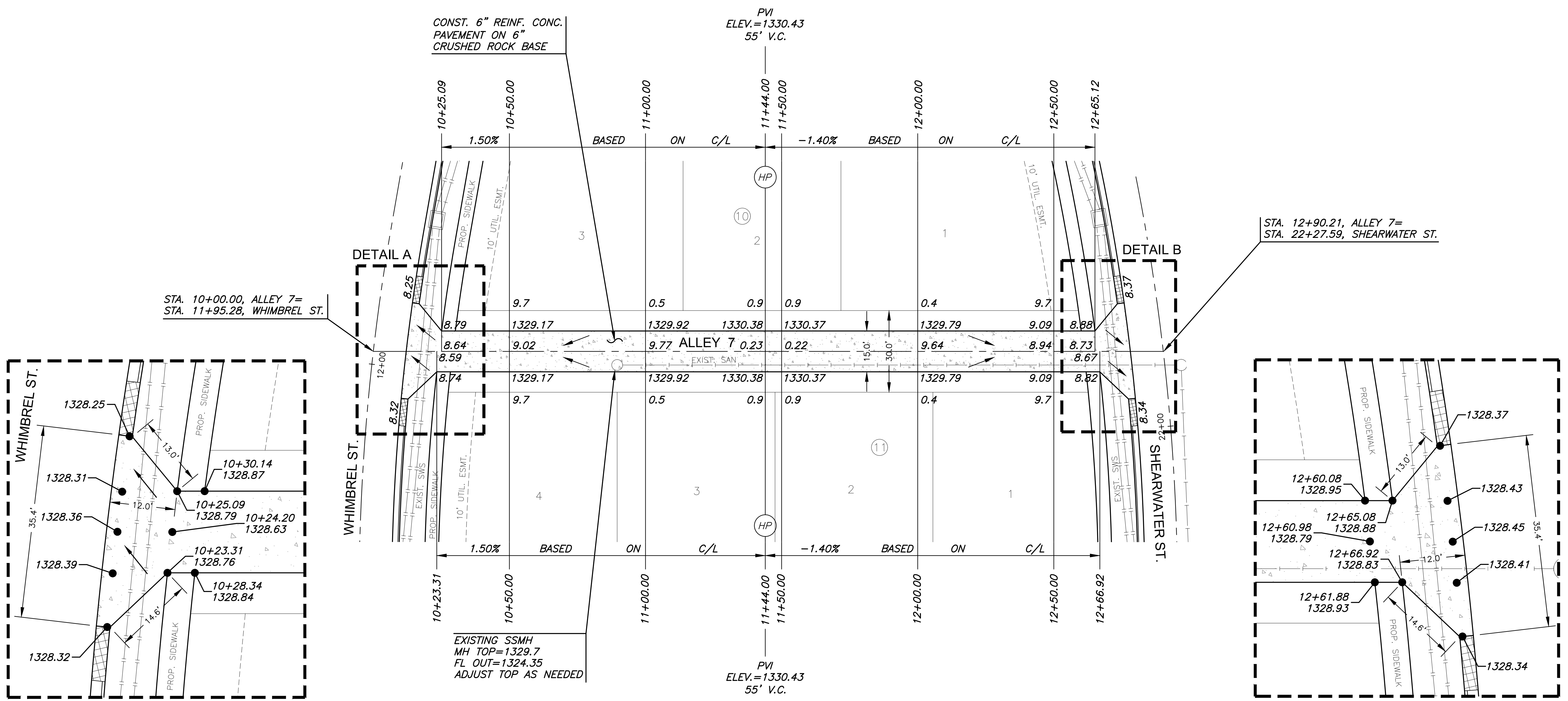
A DETAIL SCALE: 1" = 10'
