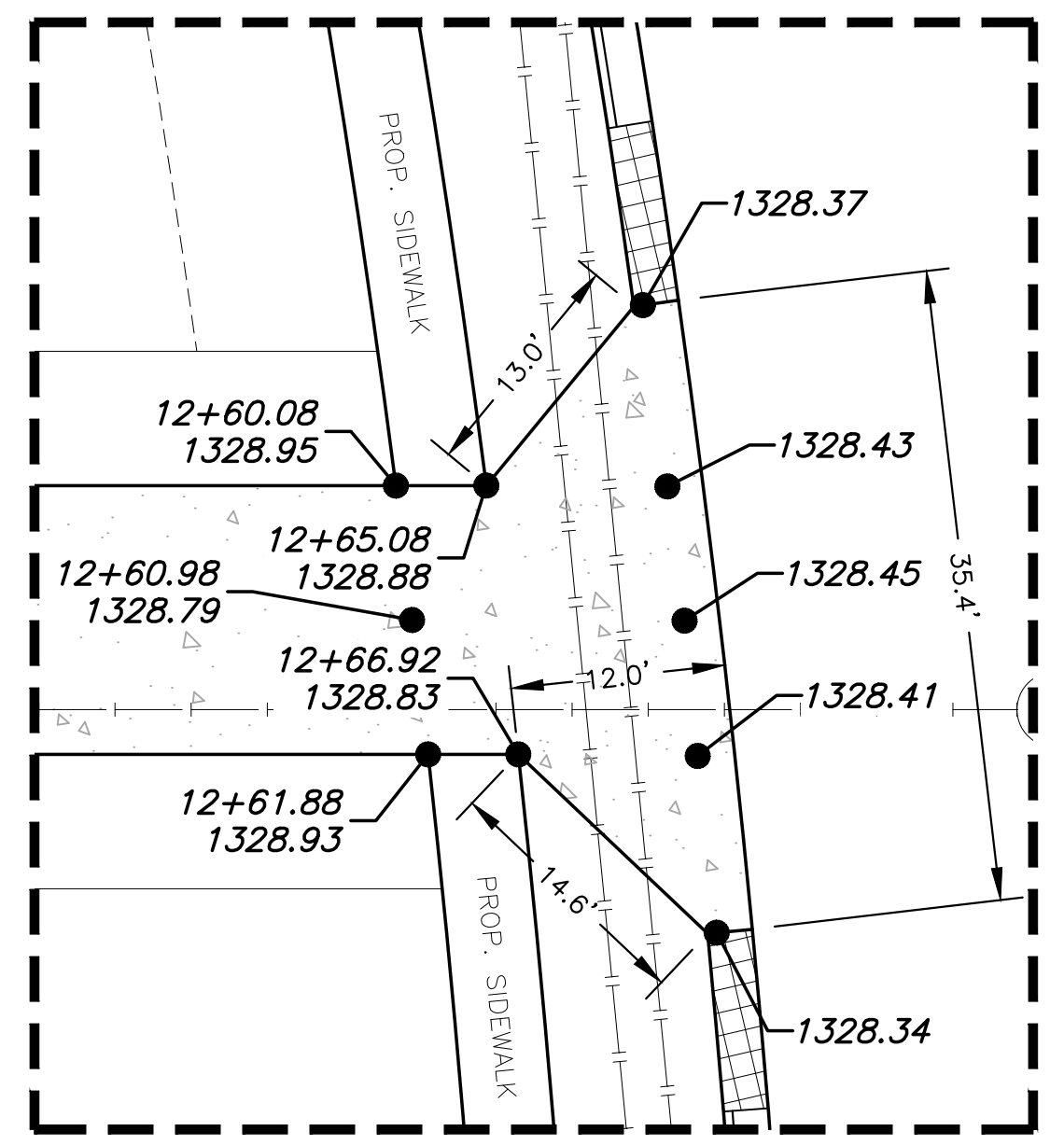
B DETAIL SCALE: 1" = 10'
