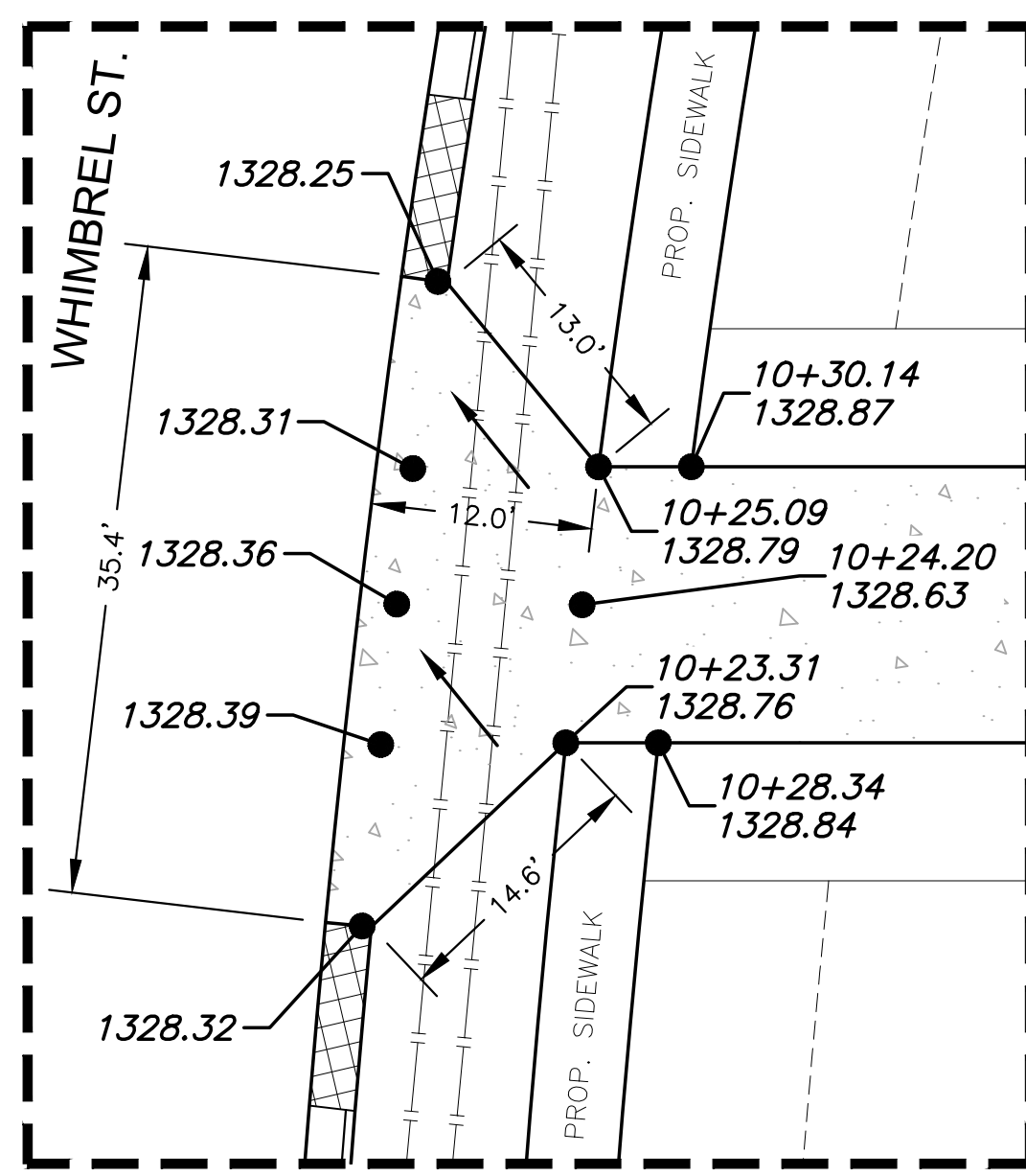
A DETAIL SCALE: 1" = 10'
