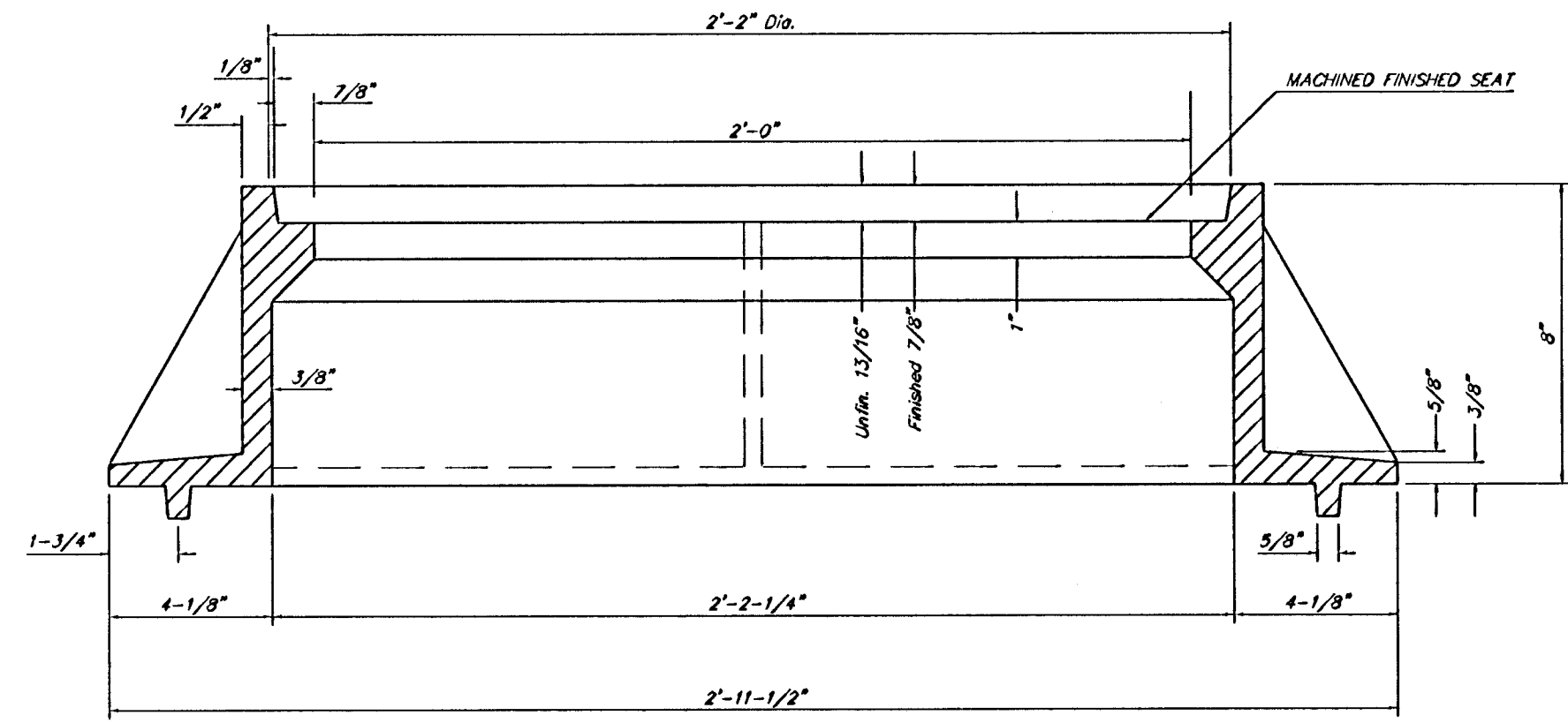
SECTION A-A
