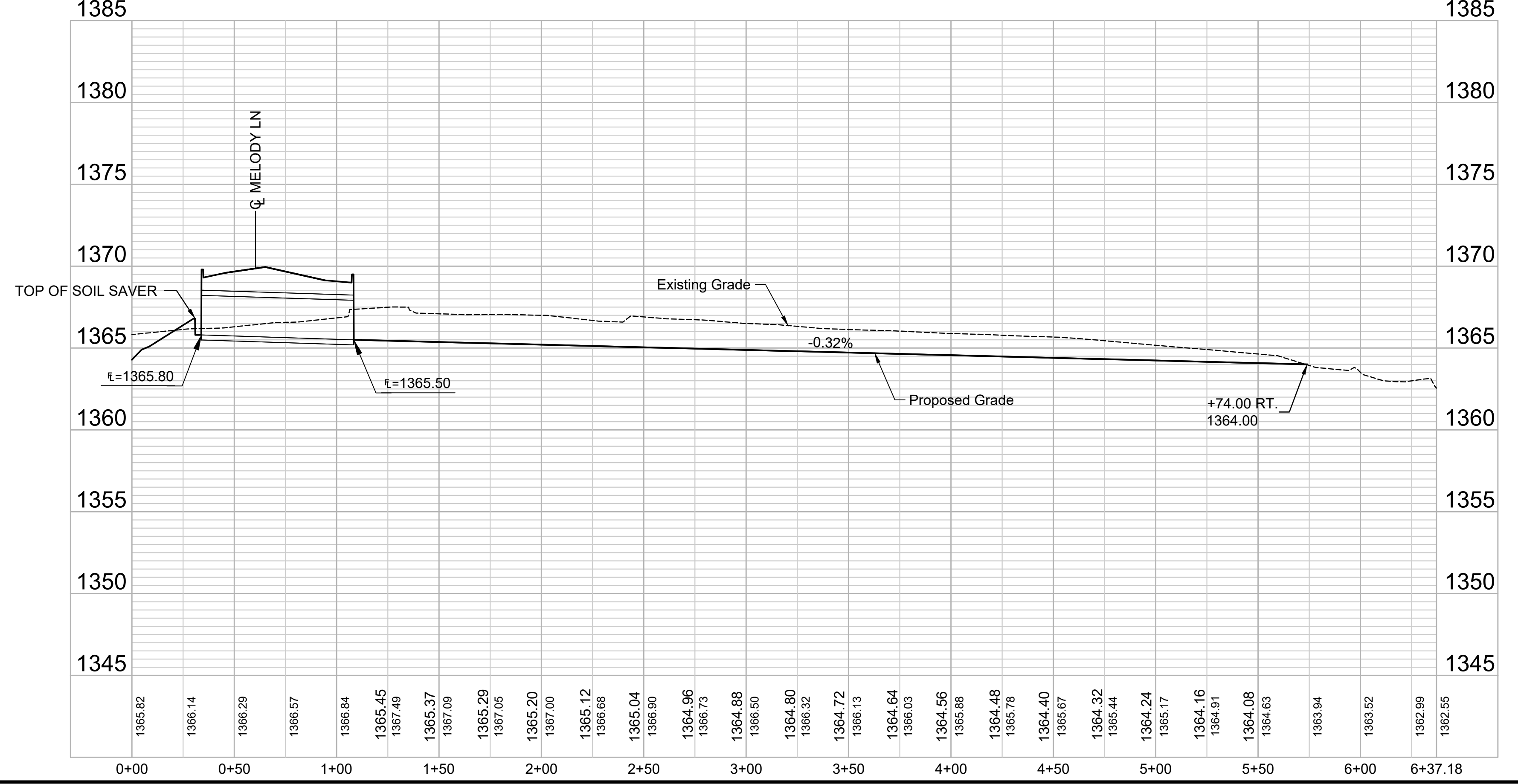
DITCH SECTION A-A
