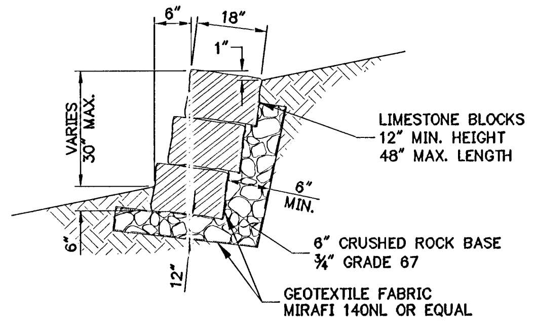
TYPE "B" WALL SCALE: N.T.S.
