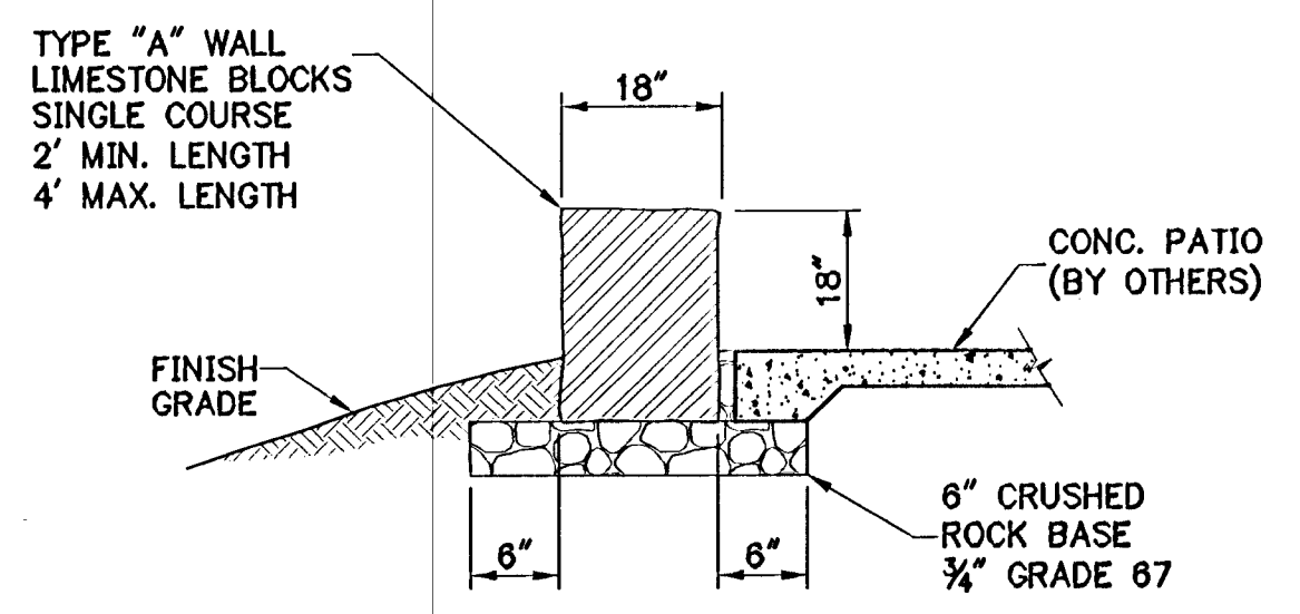
A C1.1/C1.1 PATIO WALL DETAIL SCALE: N.T.S.
