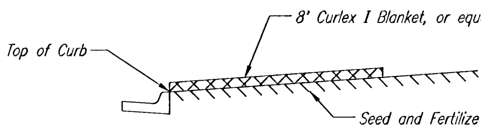
SECTION A-A
