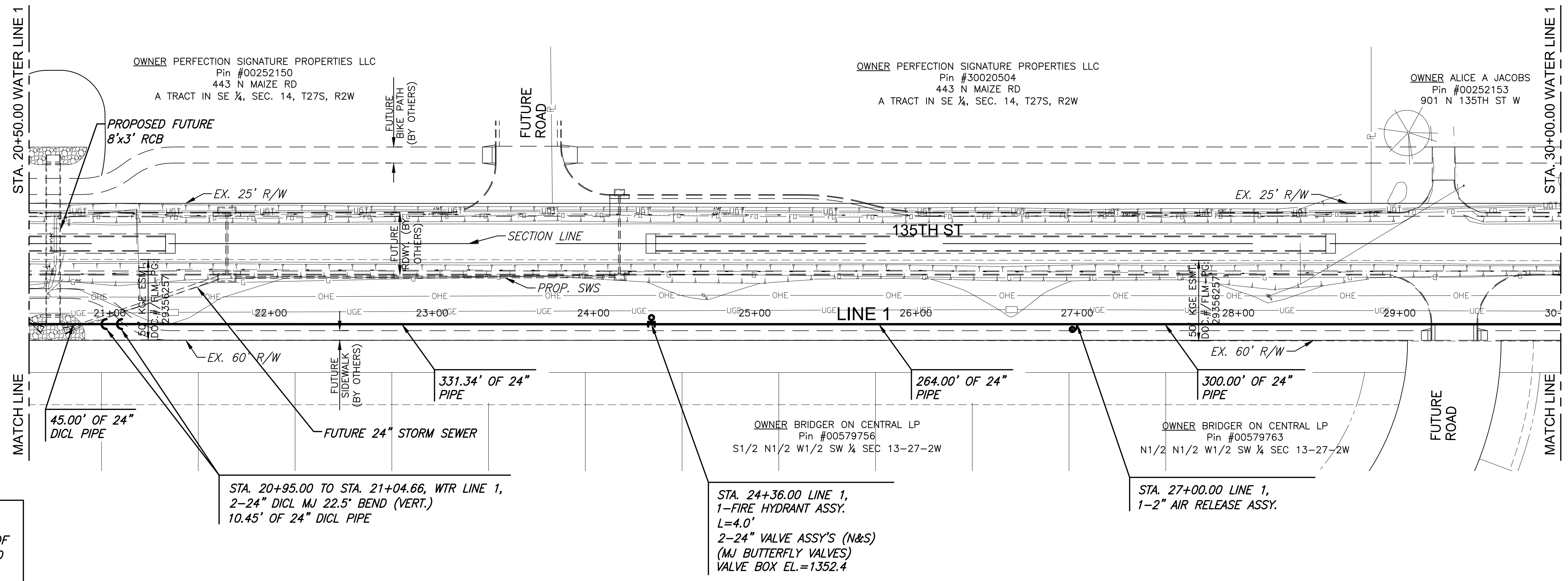
PLAN WTR LINE 1 (CONT.) PROFILE WTR LINE 1 (CONT.)
