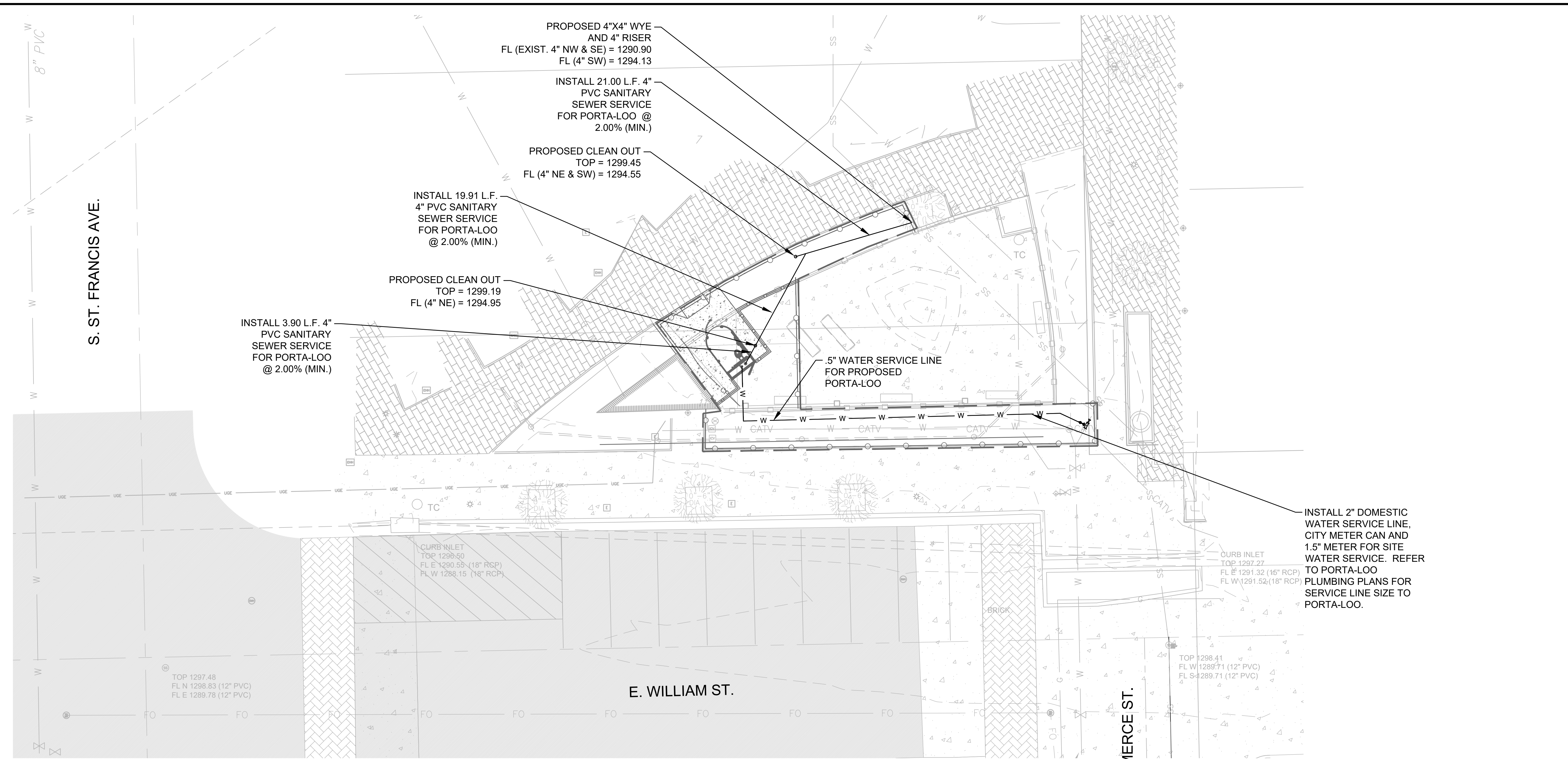
A1 UTILITY PLAN SCALE: 1" = 10'
